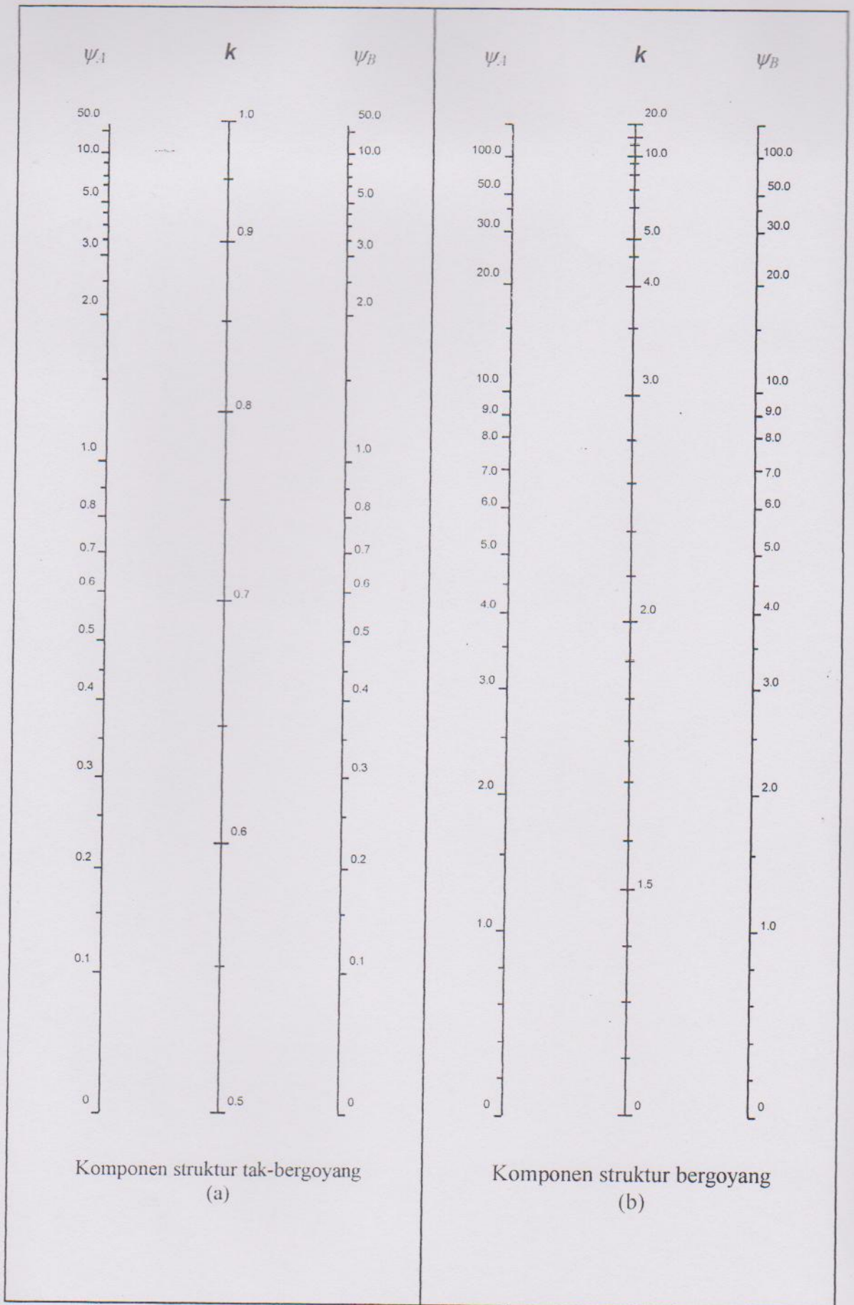
Gambar 4 Faktor panjang efektif, k
