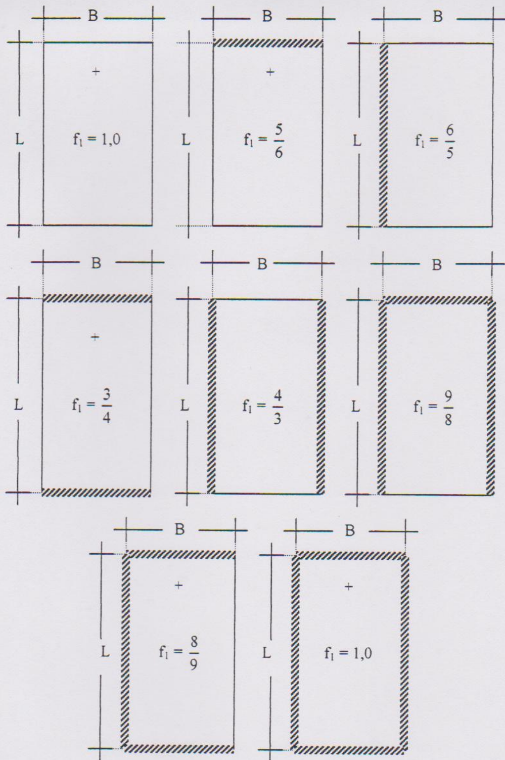
Kombinasi Perletakan Sisi Pelat dan Faktor Koreksinya, f_1 (Aswani, M.G.,1975)
