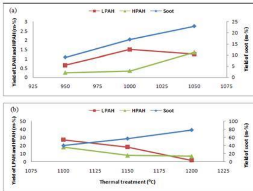
Gambar 6. Hasil perlakuan panas dari model tar sebagai fungsi suhu (a) toluena dan (b) naftalena
