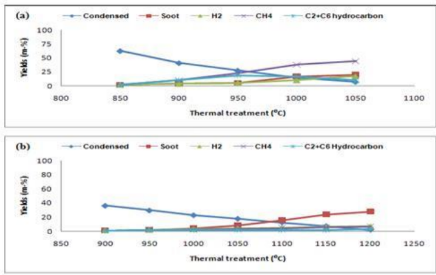
Gambar 7. Senyawa Tar yang terkandung dalam produk kental selama pengobatan termal dari model tar sebagai fungsi temperatur (a) toluena dan (b) naftalena
