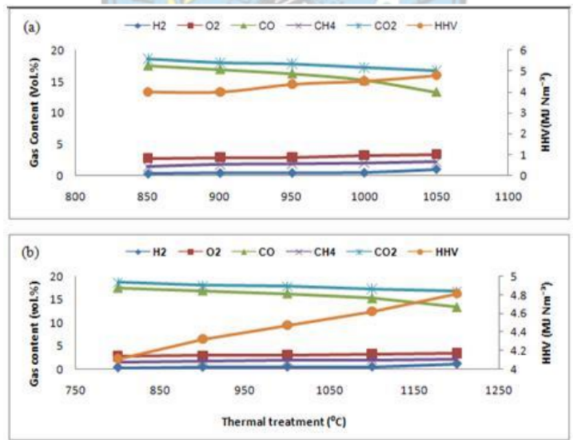
Gambar 8 : Konversi tar menjadi gas lain dan kenaikan nilai panas kalor (HHV) dengan tar model: (a) toluena dan (b) naftalena
