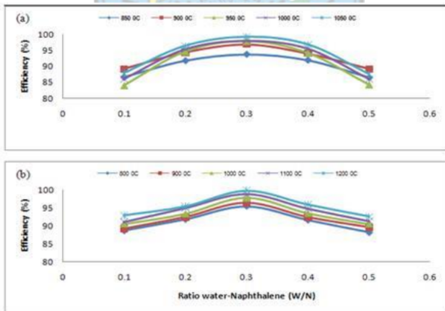
Gambar 5. Titik optimum perbandingan air-tar untuk penghapusan tar dengan model tar: (a) toluena dan (b) naftalena
