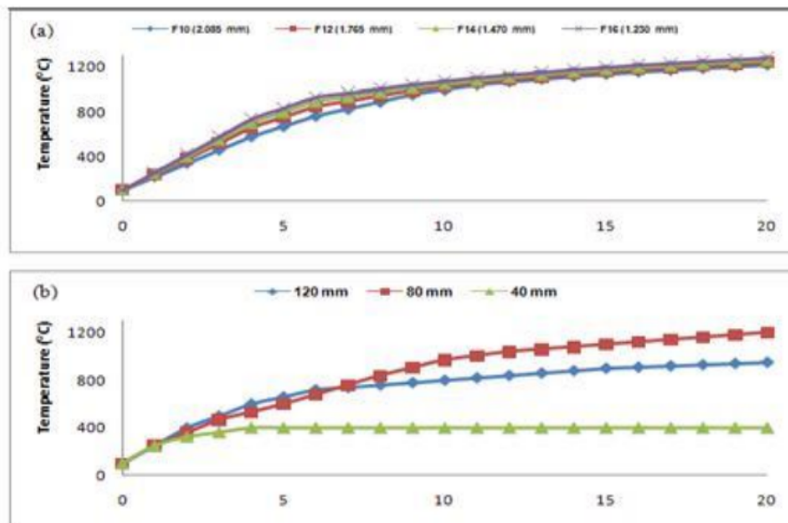
Gambar .3 profil Suhu di dalam reactor
