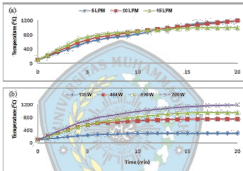
Gambar 4. profil suhu di dalam reactor (a) pengaruh laju alir gas (b) efek daya microwave
