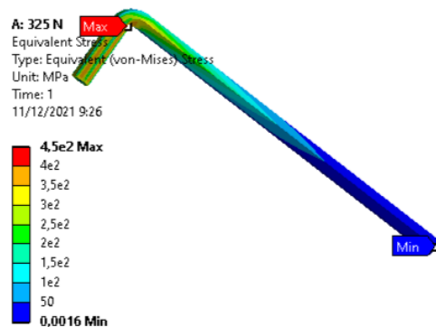
Gambar 19. Hasil Equivalent Stress Simulasi Pembebanan 325 N
