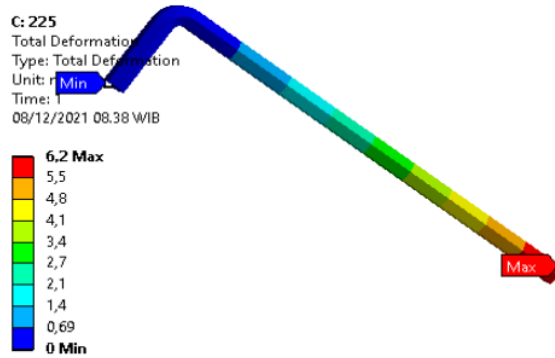
Gambar 7. Hasil Total Deformation Simulasi Pembebanan 225 N
