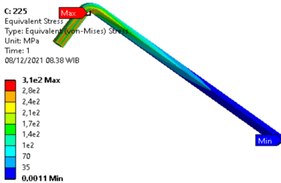
Gambar 17. Hasil Equivalent Stress Simulasi Pembebanan 225 N
