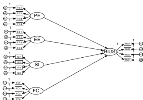
Gambar 3. Analisis Model Persamaan Struktural
