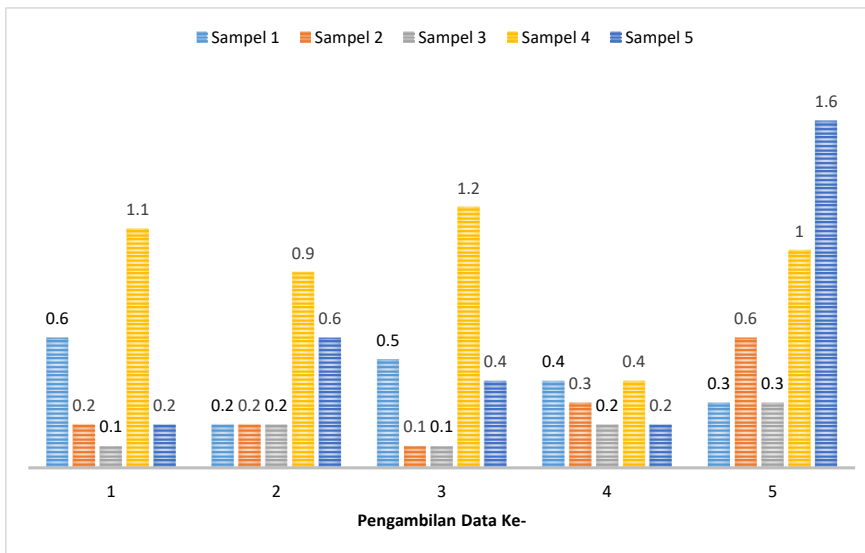
Gambar 5. Grafik Nilai Error Pada Pengujian Pengukuran Suhu
