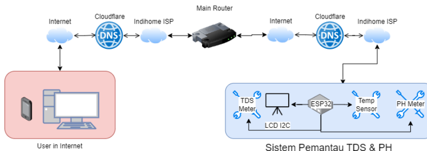
Gambar 2. Skematik Komunikasi Data Sistem Pemantauan Limbah Cair
