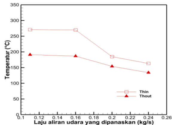
3 Gambar 6. Pengaruh laju aliran udara yang dipanaskan terhadap penurunan temperatur
