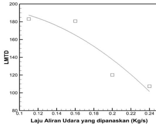
3 Gambar 5. Pengaruh laju aliran udara yang dipanaskan terhadap LMTD
