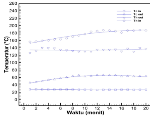
Gambar 3. Pola distribusi temperatur
