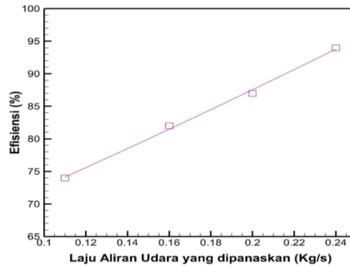
Gambar 9. Pengaruh laju aliran udara yang dipanaskan terhadap efisiensi
