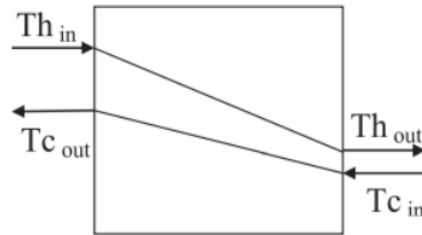
Gambar 4. Skema LMTD
