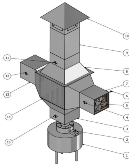
Gambar 1. Skema pengujian pengering dengan biomassa
