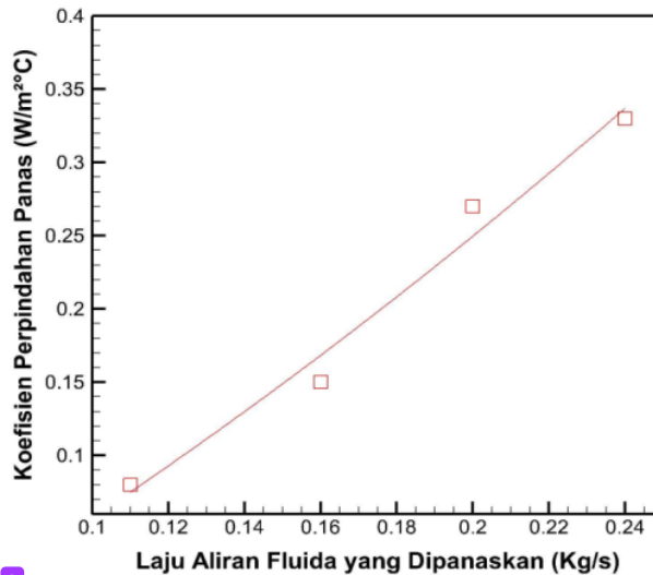
Gambar 8. Pengaruh laju aliran udara yang dipanaskan terhadap koefisien perpindahan panas
