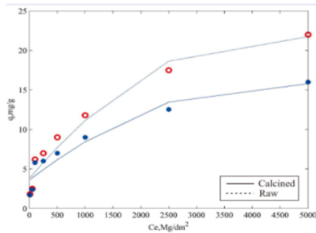
Gambar 4. Isotherm Adsorpsi Cu(II) Dari Lempung Bontang
