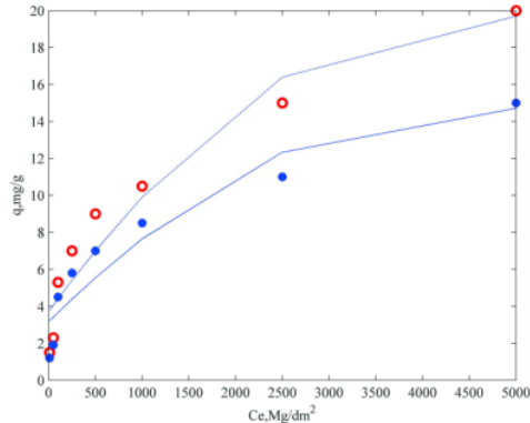
Gambar 6. Isoterm Adsorpsi Mn(II) Dari Lempung Bontang
