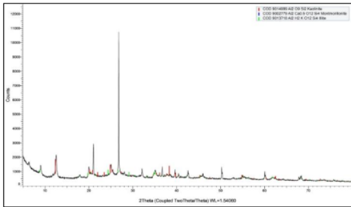
Gambar 1. Pola XRD lempung Bontang sebelum aktivasi
