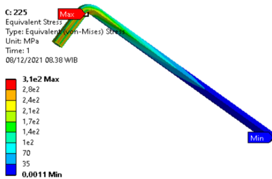
Gambar 17. Hasil Equivalent Stress Simulasi Pembebanan 225 N
