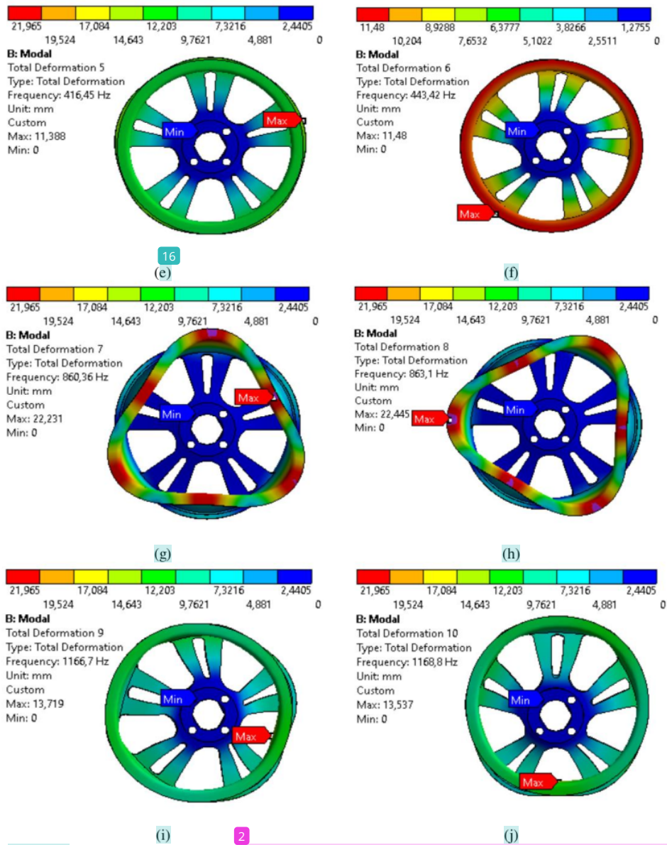
Gambar 2. Mode getar velg ring 16 (a) pertama, (b) kedua, (c) ketiga, (d) keempat, (e) kelima, (f) keenam, (g) kedelapan, (h) kesembilan, (j) kesepuluh.
