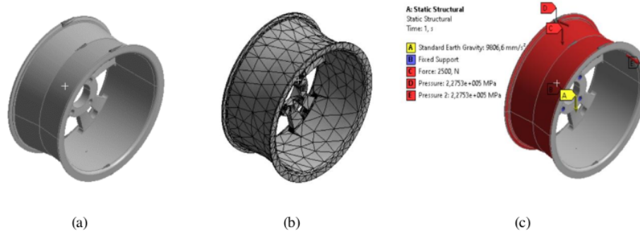
Gambar 1. Tahapan simulasi pemodelan frekuensi natural velg mobil ring 16 (a) desain pemodelan velg ring 16 menggunakan software 3D, (b) pembagian domain komputasi, (c) initial condition velg mobil ring 16.
