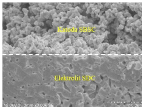
Gambar 6: Penampang spesimen sel simetris
