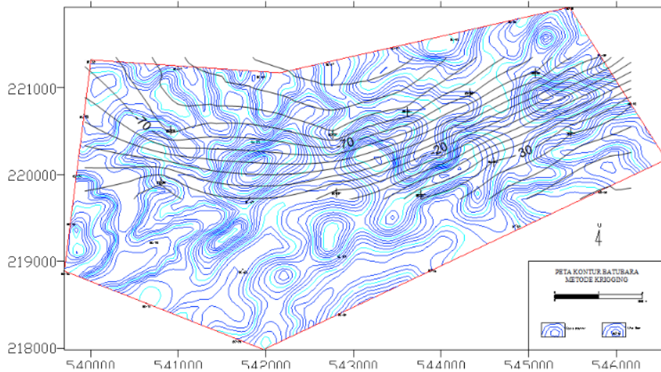
Gambar 2. Kontur Lapisan Batubara Metode Triangulasi
