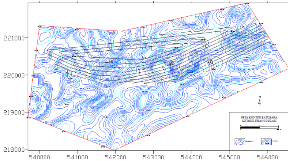
Gambar 1. Kontur Lapisan Batubara Metode Triangulasi
