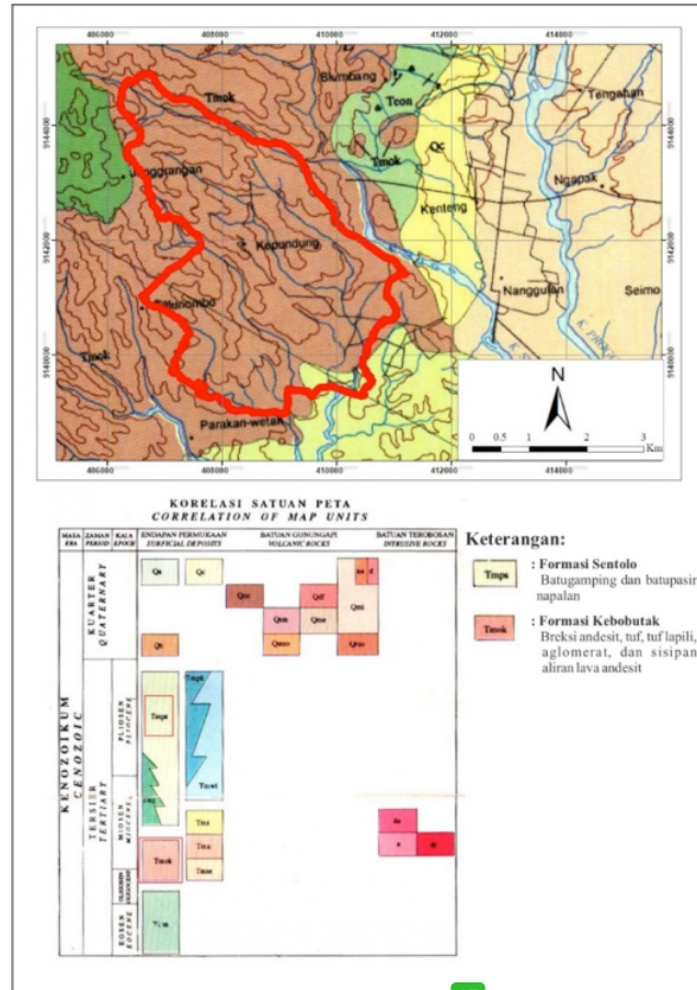
Gambar 2. Stratigrafi regional daerah penelitian
