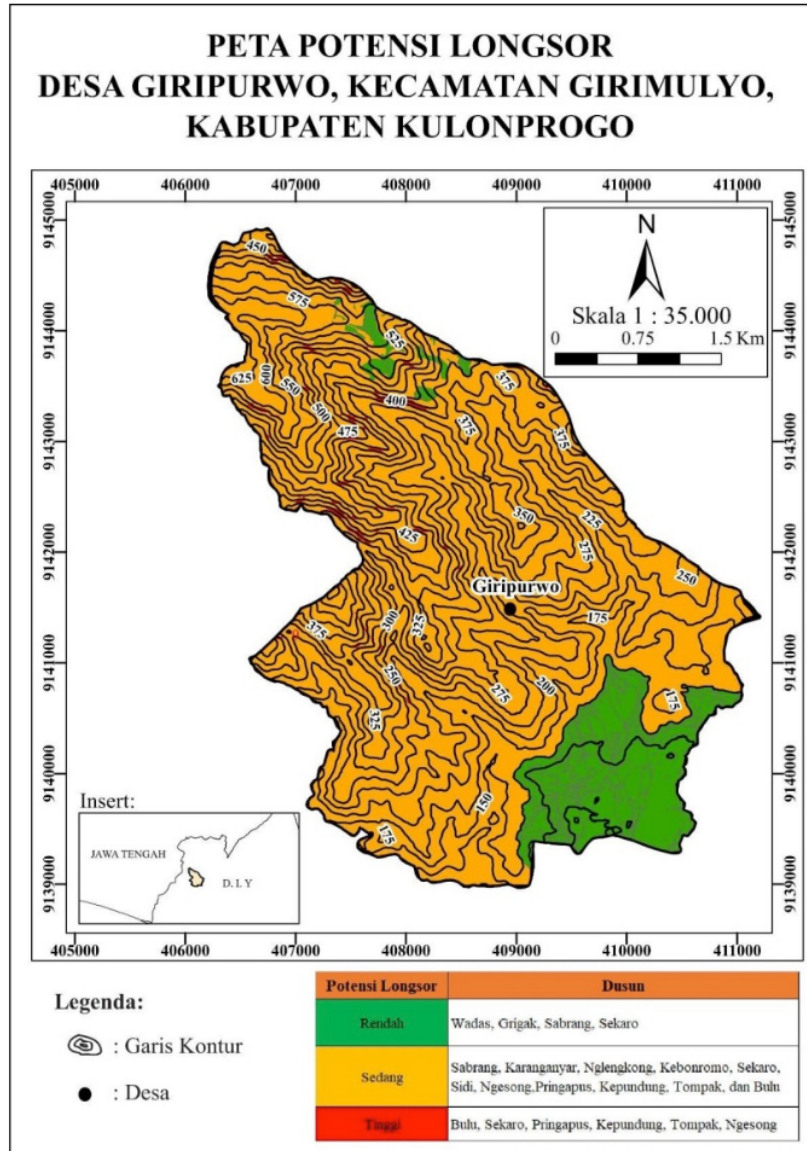
Gambar 11. Peta potensi longsor Desa Giripurwo
