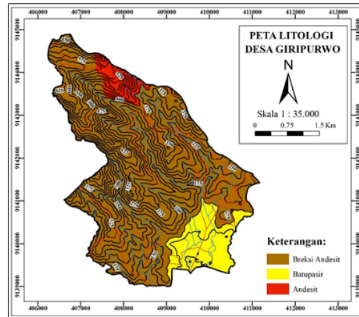
Gambar 8. Peta penyebaran litologi Desa Giripurwo
