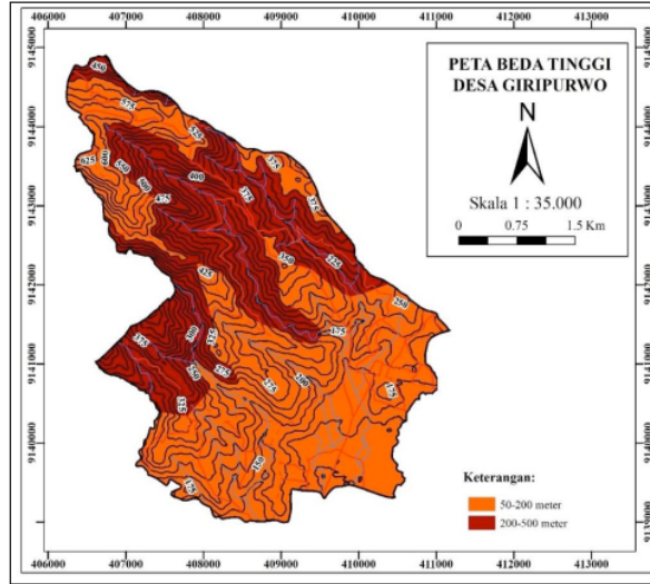
Gambar 4. Peta beda tinggi Desa Giripurwo
