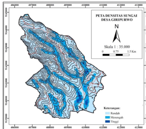
Gambar 10. Peta densitas sungai Desa Giripurwo
