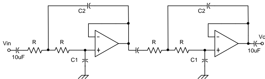
Gambar 5. Rangkaian dasar LPF 4 KHz – 0,5 KHz orde 4
