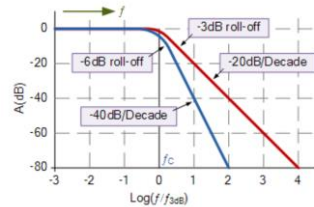
Gambar 2. Tanggapan frekuensi LPF orde 1 dan orde 2
