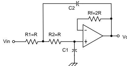
Gambar 1. Rangkaian LPF orde 2
