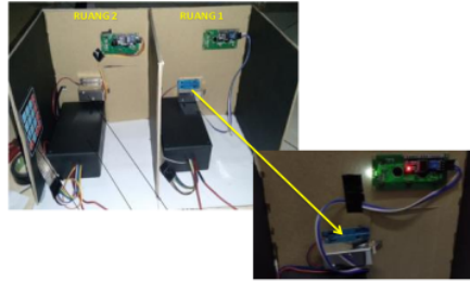
Gambar 8. Selenoid doorlock mengunci
