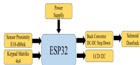
Gambar 2. Diagram blok perancangan sistem elektrik
