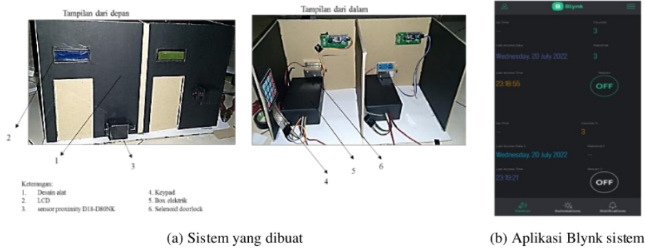
Gambar 5 Hasil rancang bangun sistem
