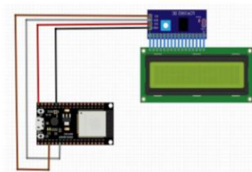
Rangkaian LCD+I2C ke ESP32
