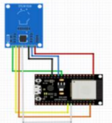
Rangkaian MFRC522 RFID reader
