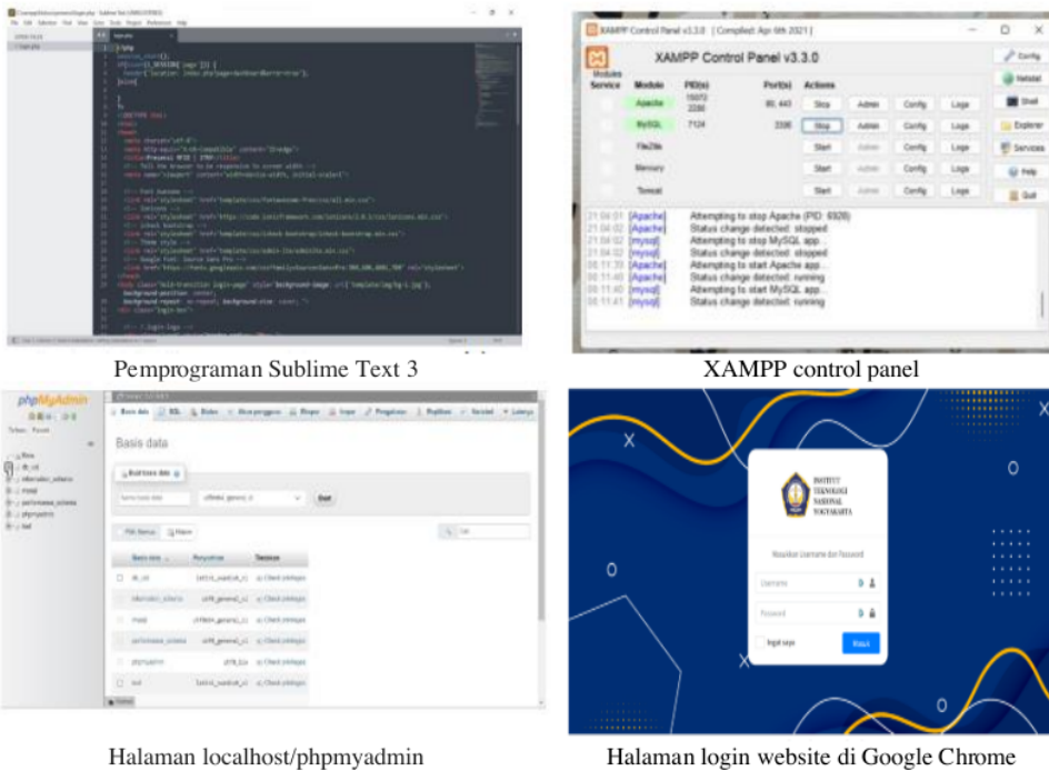
Gambar 3. Perancangan Software
