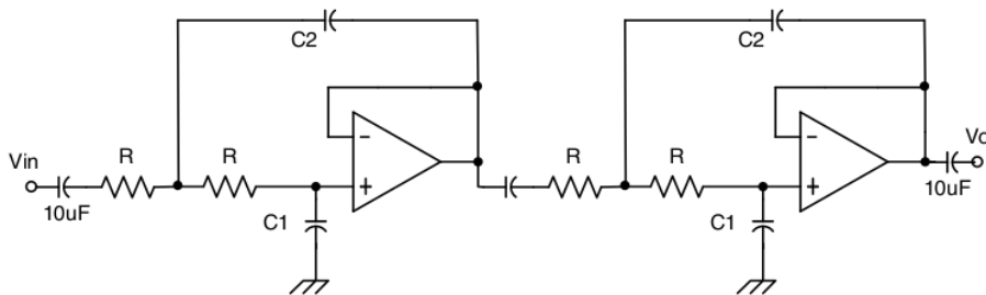
Gambar 5. Rangkaian dasar LPF 4 KHz – 0,5 KHz orde 4
