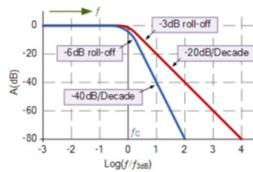
Gambar 2. Tanggapan frekuensi LPF orde 1 dan orde 2
