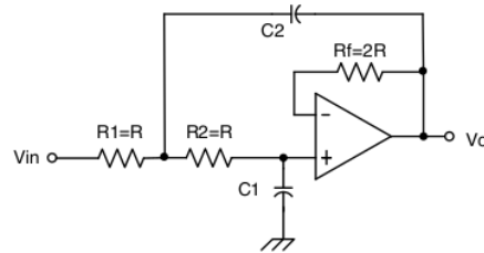
Gambar 1. Rangkaian LPF orde 2
