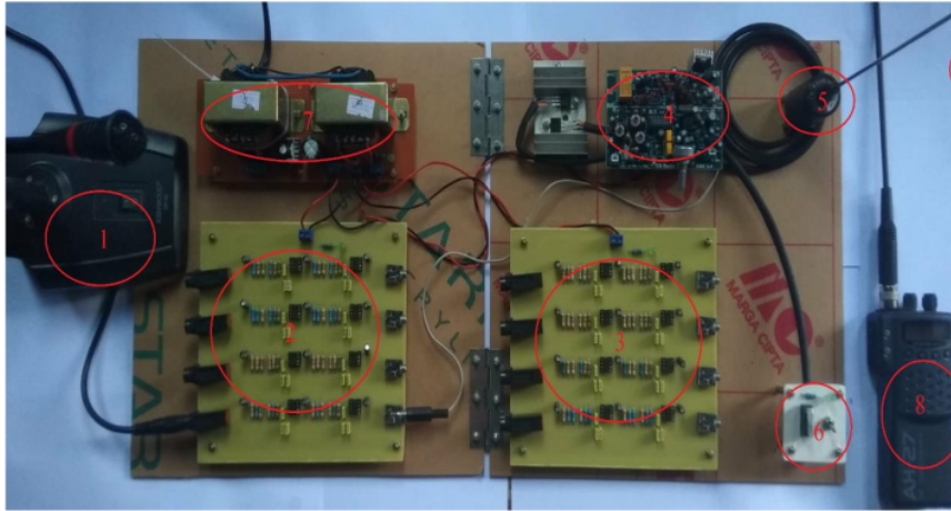
Gambar 6. Hasil perancangan perangkat keras
