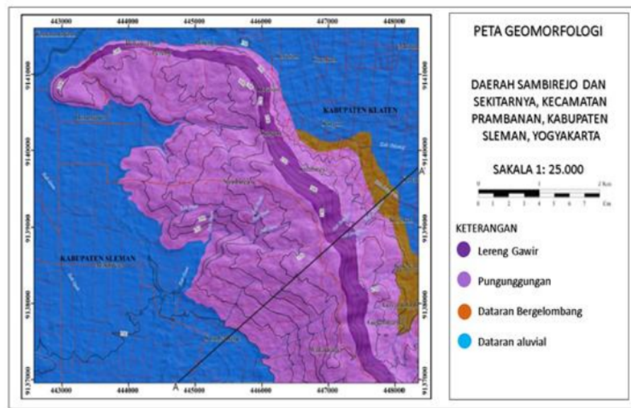
Gambar 2. Peta Geomorfologi.
