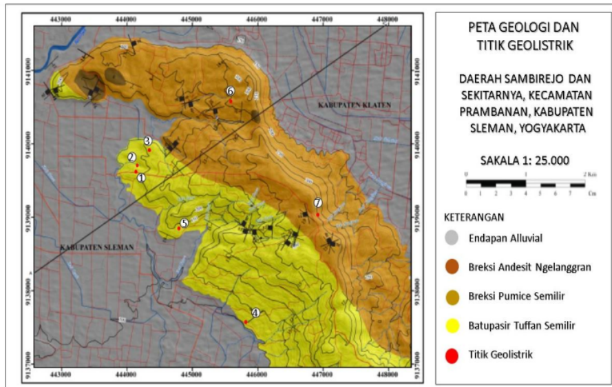
Gambar. 3. Peta Geologi.
