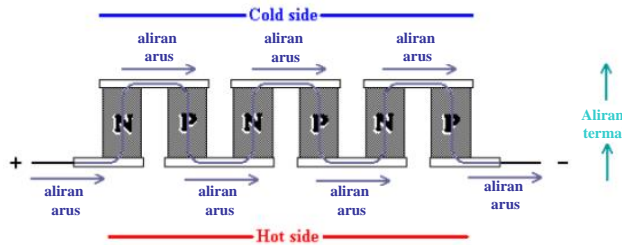
Gambar 2 Elemen thermoelectric yang tersusun seri
