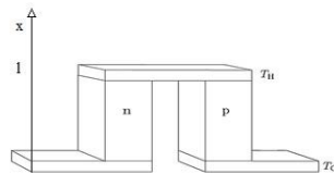
Gambar 1 Bentuk dasar divais termoelektrik ( thermocouple )
