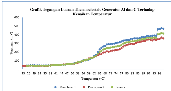
Gambar 10. Grafik hasil pengukuran tegangan luaran terhadap kenaikan temperatur
