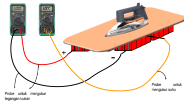
Gambar 7. Ilustrasi proses pengukuran tegangan luar dan temperatur
