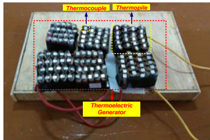
Gambar 8. Thermoelectric Generator Al dan C
