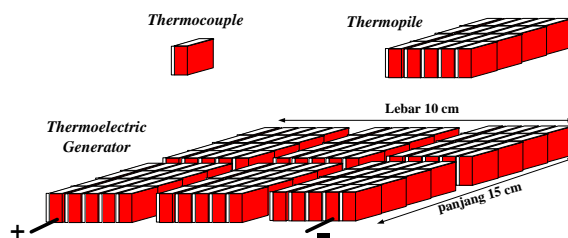
Gambar 6. Thermoelectric Generator dari Aluminium dan isi pensil
