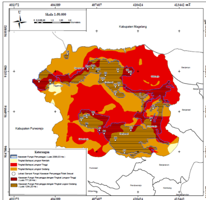
Gambar 4. Zona potensi kerawanan longsor pada lahan dengan fungsi kawasan penyangga
