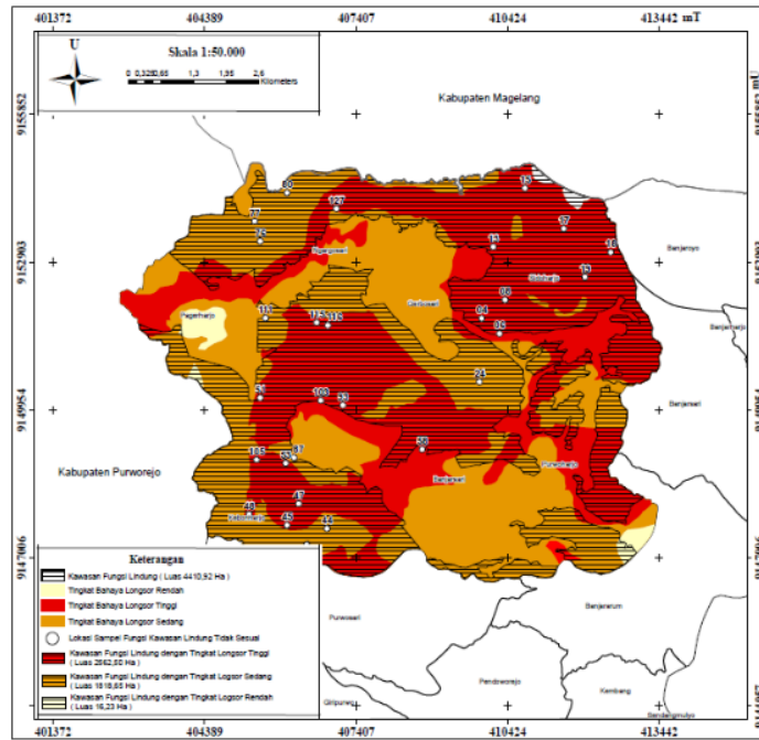
Gambar 3. Zona potensi kerawanan longsor pada lahan dengan fungsi kawasan lindung
