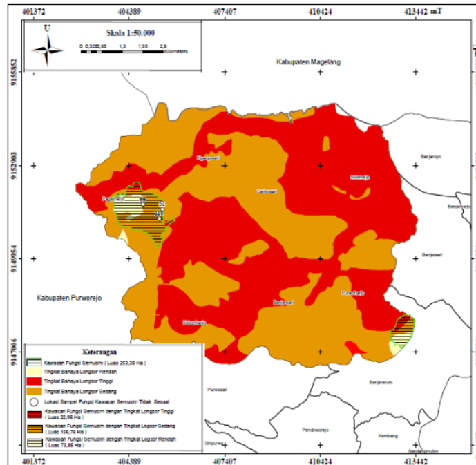
Gambar 5. Zona potensi kerawanan longsor pada lahan dengan fungsi kawasan budidaya tanaman semusim
