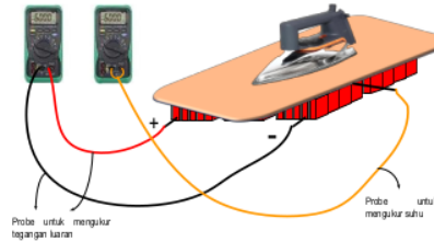
Gambar 7. Ilustrasi proses pengukuran tegangan luaran dan temperatur
