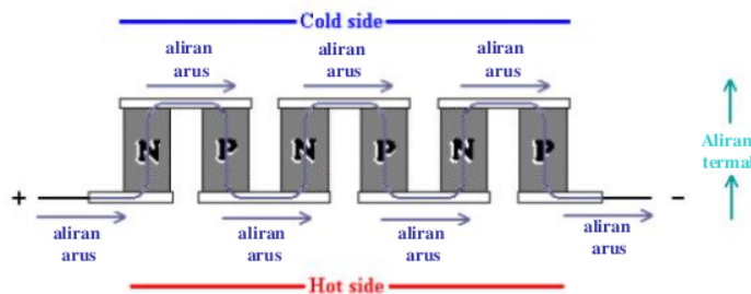
Gambar 2 Elemen thermoelectric yang tersusun seri
