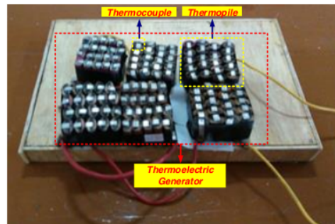
Gambar 8. Thermoelectric Generator Al dan C
