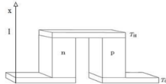
Gambar 1 Bentuk dasar divais termoelektrik ( thermocouple )
