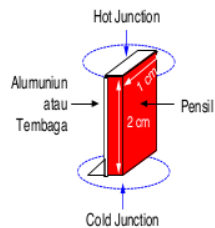
Gambar 5. Termokopel jenis aluminium dan karbon (pensil)
