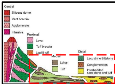
Gambar 10 . Model fasies gunungapi, lokasi penelitian berada pada fasies Medial .( Bogie & Mackenzie, 1998).
