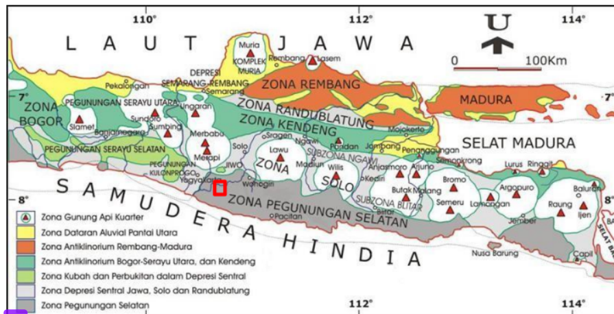
Gambar 2. Fisiografi bagian Tengah dan Timur Pulau Jawa (Van Bemmelen, 1949 dalam Hartono, 2010) . Kotak merah daerah penelitian.
