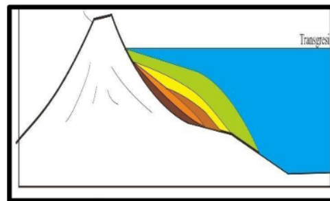
Gambar 15. Lingkungan Pengendapan Satuan Batulanau
