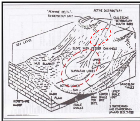
Gambar 11. Rekonstruksi Kipas Bawah Laut Walker (1984).
