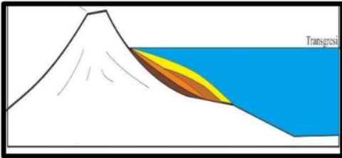
Gambar 14. Lingkungan Pengendapan Satuan Batupasir
