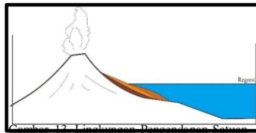
Gambar 13. Lingkungan Pengendapan Satuan
