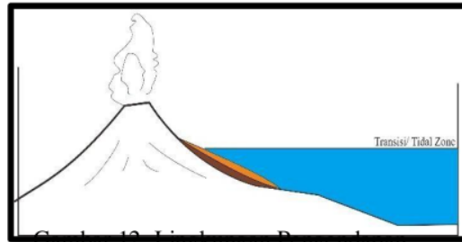
Gambar 12. Lingkungan Pengendapan
