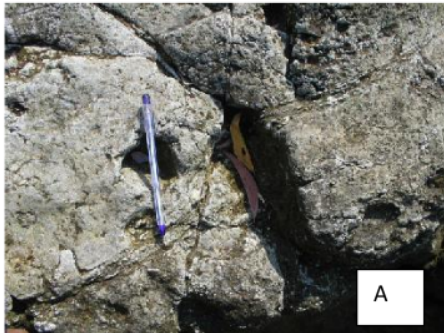
Gambar 5. A) Kenampakan sesar minor N110°E/80° memotong kekar N175°E/65°, foto menghadap ke barat laut. B) breksi sesar di pertemuan Kali Opak dan kali Oyo.
