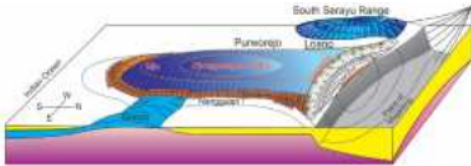
Gambar 2. Bentuk secara landscape Oblong dome terdiri dari sisa Gunung Gajha kuno, Gunung Berapi Menoreh, dan Gunung Idjo (dimodifikasi oleh van Bemmelen 1949, dalam Hartono 2017).
