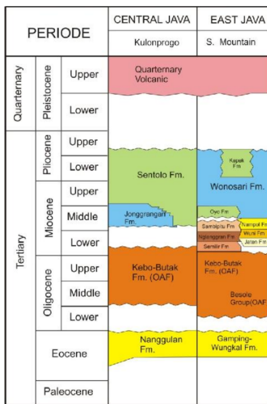
Gambar 2. Stratigrafi regional Yogyakarta dan sekitarnya (Surono, dkk., 1992 dan Rahardjo, dkk., 1995)
