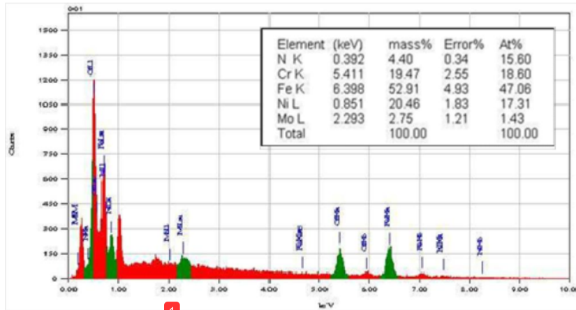
Gambar 7. Hasil uji EDS SS 316L setelah proses nitridasi plasma pada temperatur 550°C.
