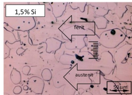
Gambar 4. Struktur mikro paduan Fe-7,5Al-5Mn-Si
