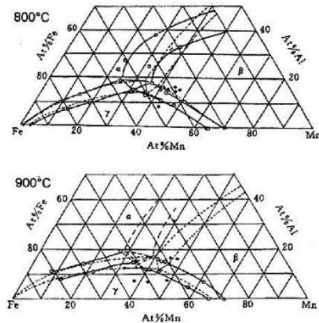
Gambar 3. Diagram Fasa Ternary Fe-Al-Mn (Chao dan Liu, 2002)
