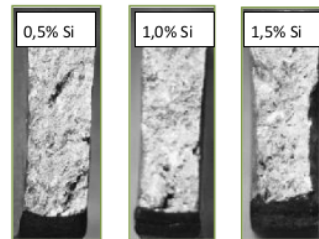
Gambar 6. Permukaan patah specimen uji impak
