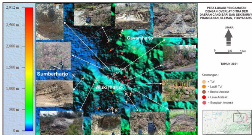
Gambar 3. Peta Lokasi Pengamatan dengan Sebagian Foto Singkapan yang Menguatkan Adanya Gunung Api Purba pada Daerah Penelitian
