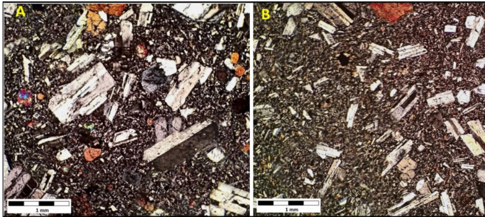
Gambar 6. Kenampakan Petrografi yang Diambil pada Lava (Lokasi C20) Menunjukkan Adanya Tekstur Pilotaxitic dengan Nama Batuan Pilotaxitic Piroxene Andesite (A) dan Kenampakan Petrografi yang Diambil pada Bongkah (Lokasi C22) dengan Nama Batuan Piroxene Andesite (B)
