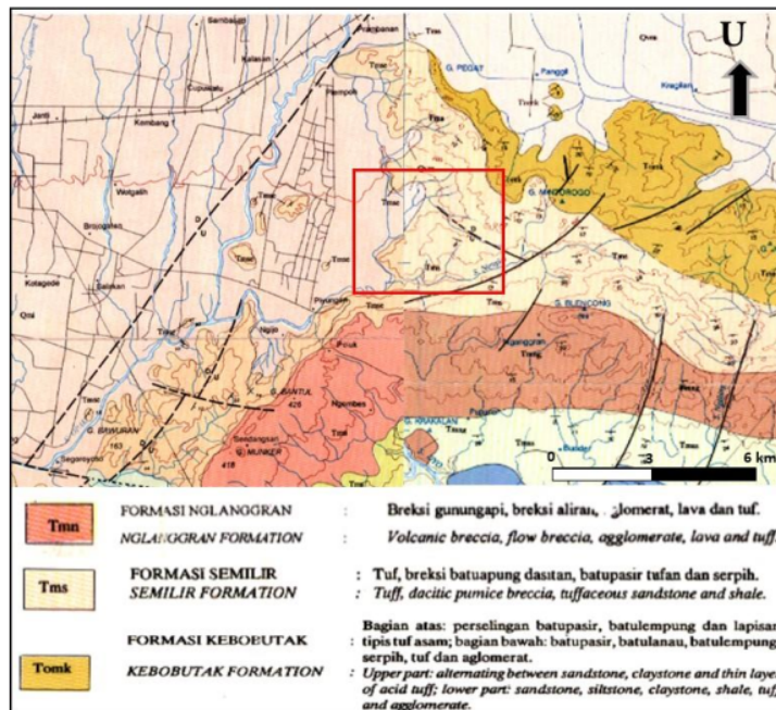
Gambar 2. Peta Geologi Regional Daerah Penelitian yang Masuk pada Lembar Surakarta-Giritronto [1] dan Lembar Yogyakarta [2] dengan Lokasi Penelitian Ditunjukkan Kotak Warna Merah
