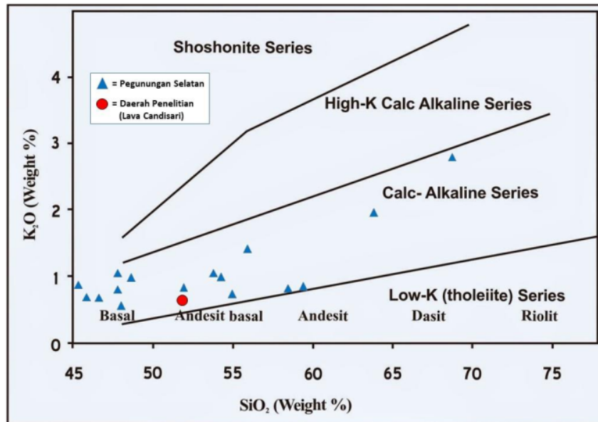
Gambar 9. Afinitas Magma Pembentuk Batuan pada Lava Andesit Daerah Penelitian (Candisari) Dibandingkan dengan Beberapa Batuan Beku yang Ada di Pegunungan Selatan [5]
