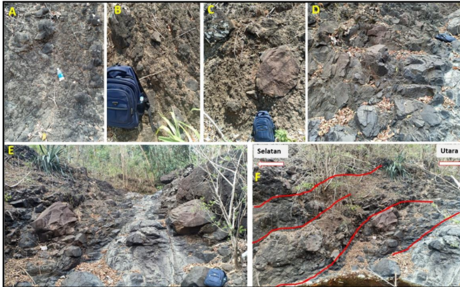
Gambar 5. Breksi Andesit yang Mengandung Bom dan Blok Gunung Api (A, B, C), Lava Andesit yang Membereksi ( Autobreccia ) (E) dan Perkiraan Arah Umum Aliran Lava Relatif Utara-Selatan (F)
