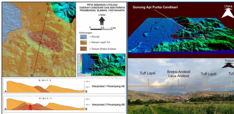
Gambar 4. Peta Geologi Sederhana Daerah Penelitian (Sebelah Kiri), Kenampakan Peta DEM secara 3D (Kanan Atas) dan Pandangan Katak Daerah Candisari dan Sekitarnya (Kanan Bawah)
