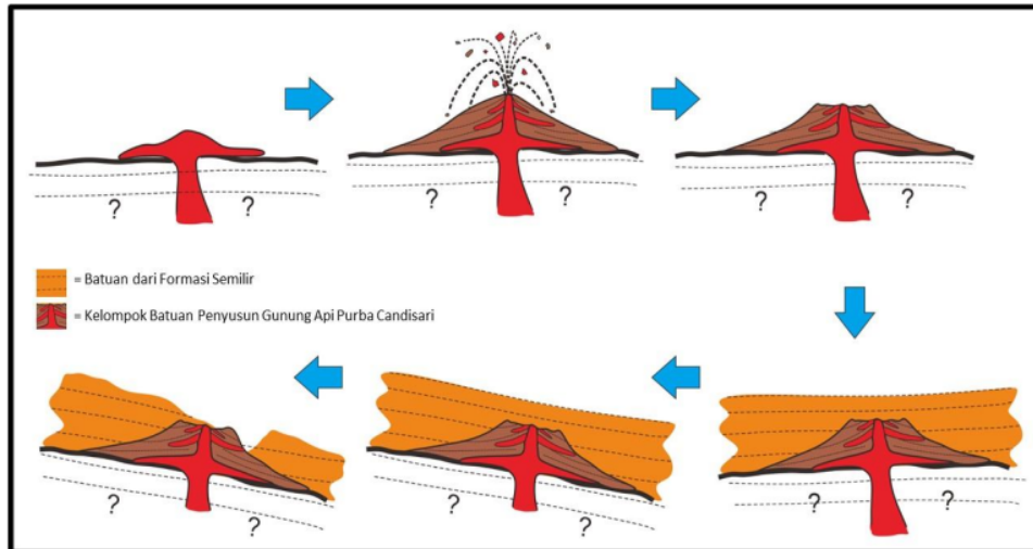
Gambar 10. Model Sederhana Pembentukan Gunung Api Purba Candisari dan Kedudukannya dengan Formasi Semilir (Tidak Dalam Skala Sebenarnya)
